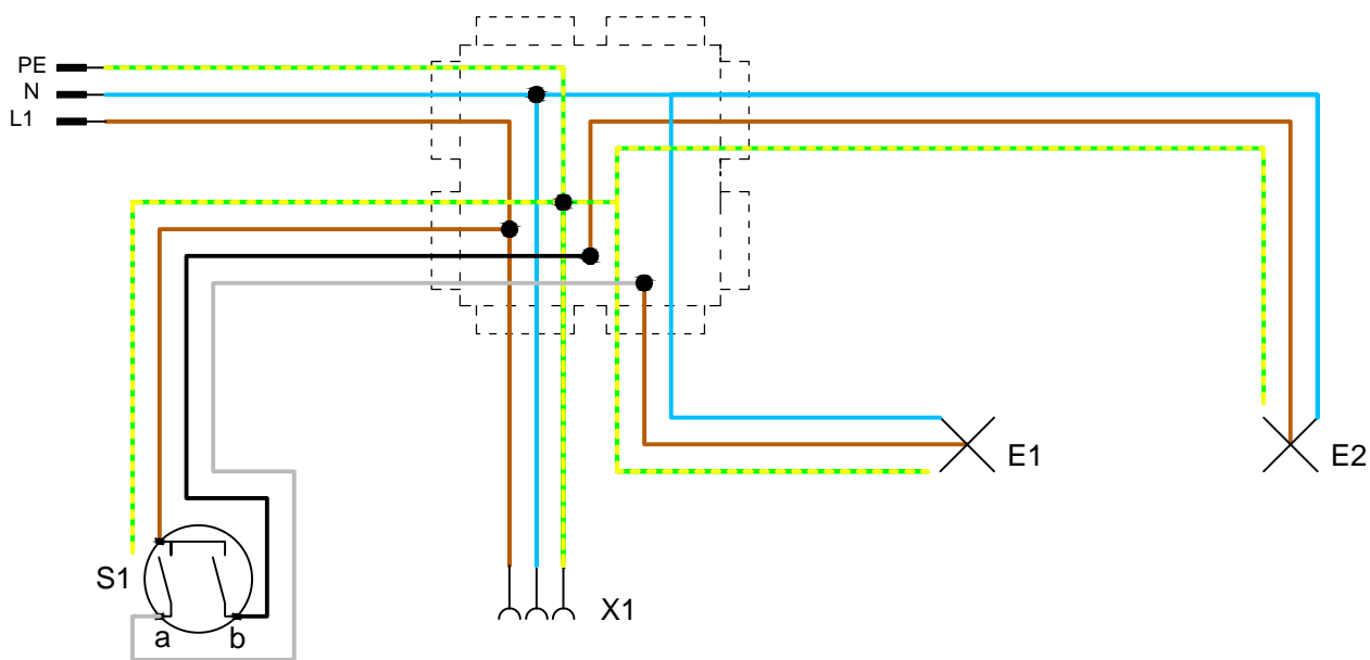
Bedradingschema
