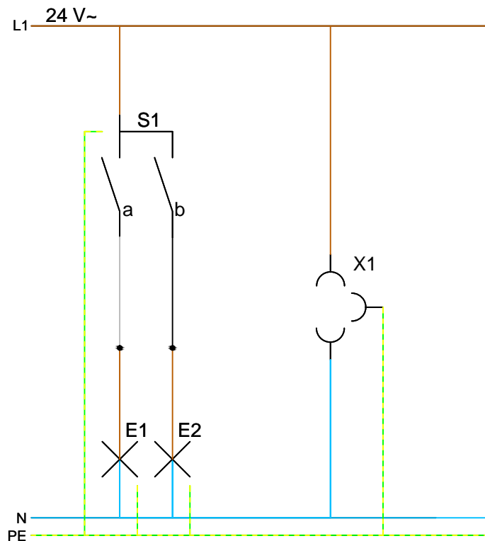
Stroomkringschema
