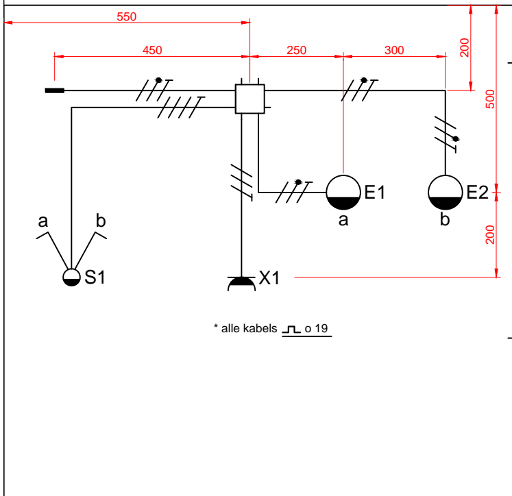
Installatieschema
